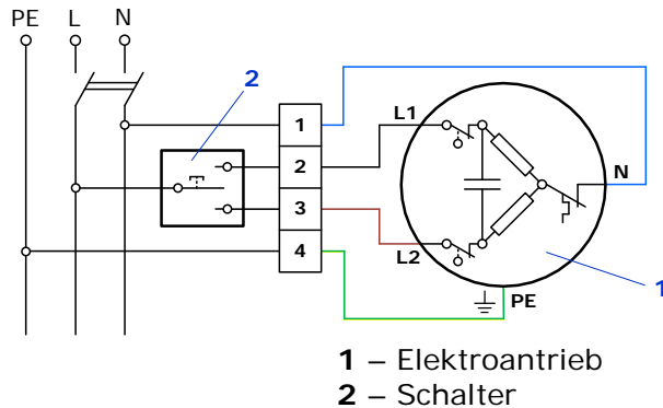
Bild 1. Elektrische Anschlüsse
